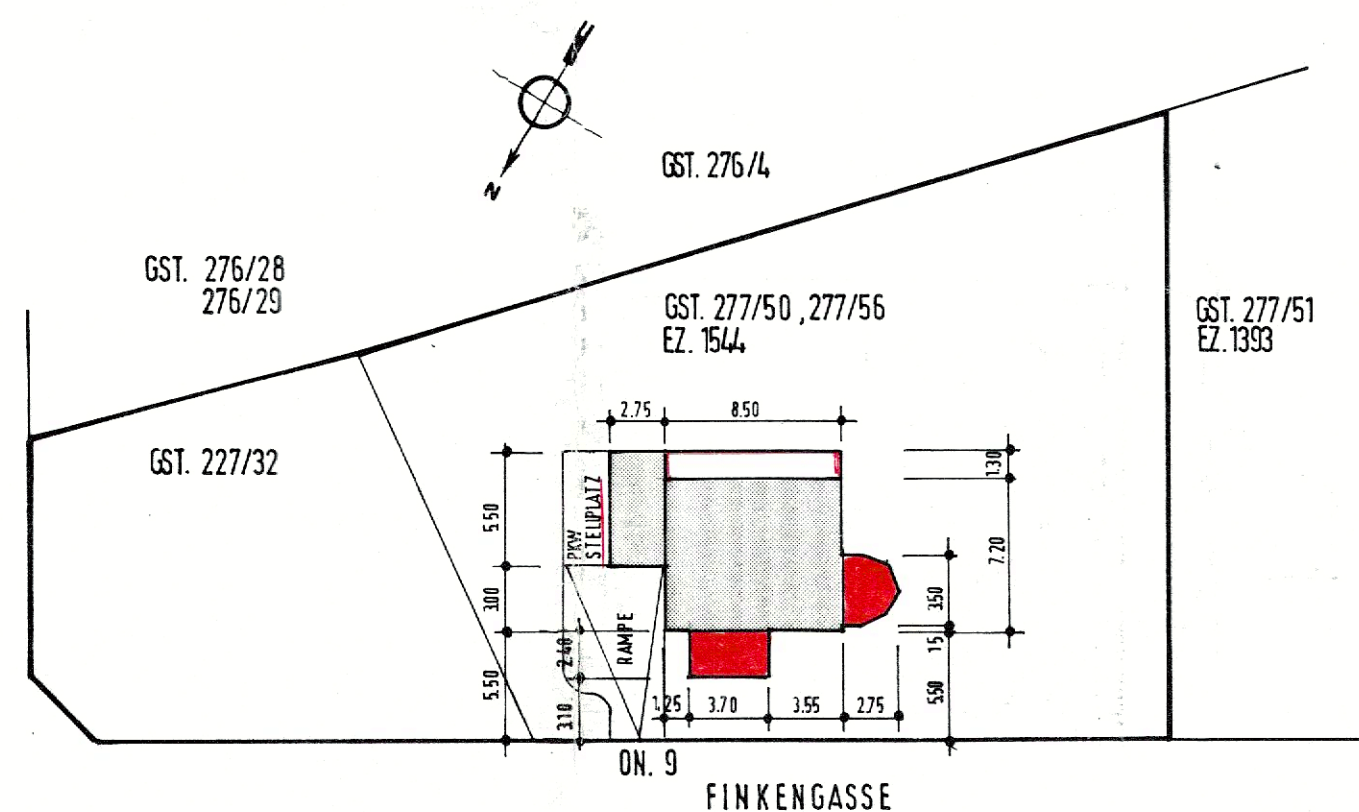
LAGEPLAN M. 1:360
