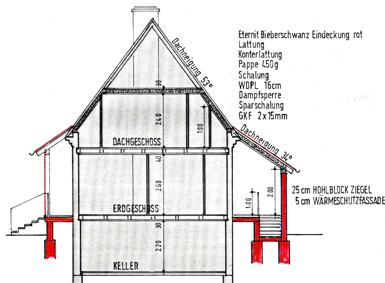
SCHNITT A-A
