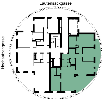
GESCHOSSPLAN
