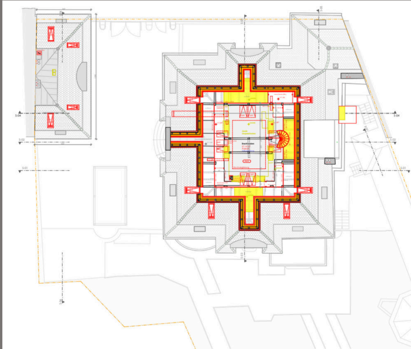
2. Dachgeschoss
