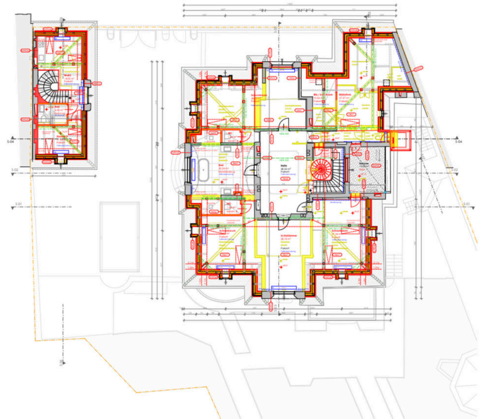
1. Dachgeschoss
