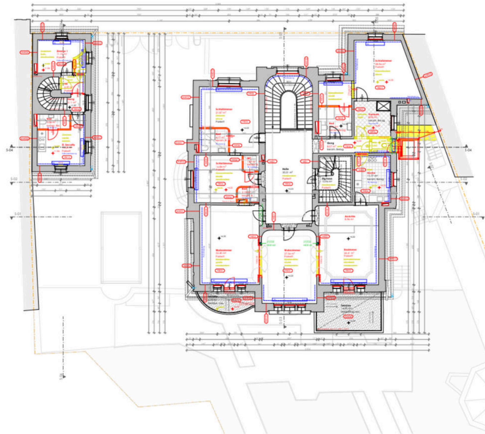
1. Obergeschoss
