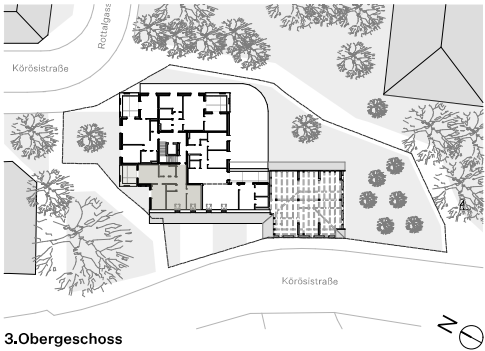
3.Obergeschoss
