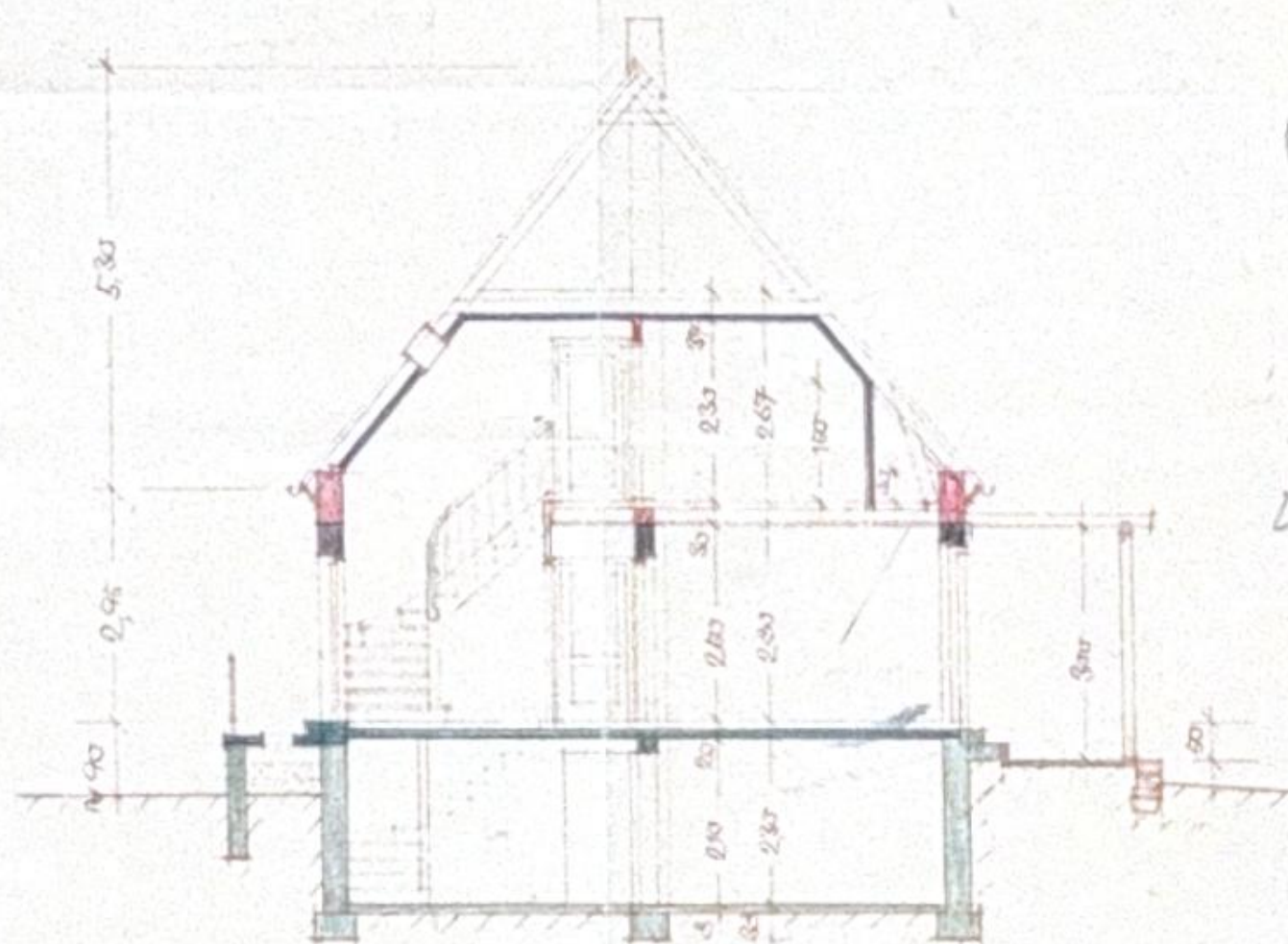
HÖHENSCHNITT
