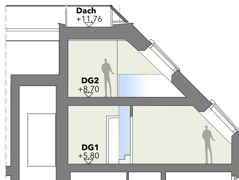
Schnitt
