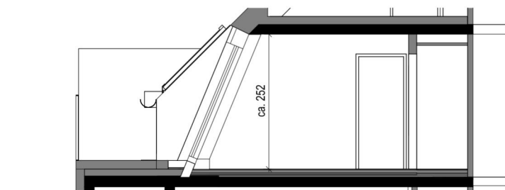
Schnitt 48.A
