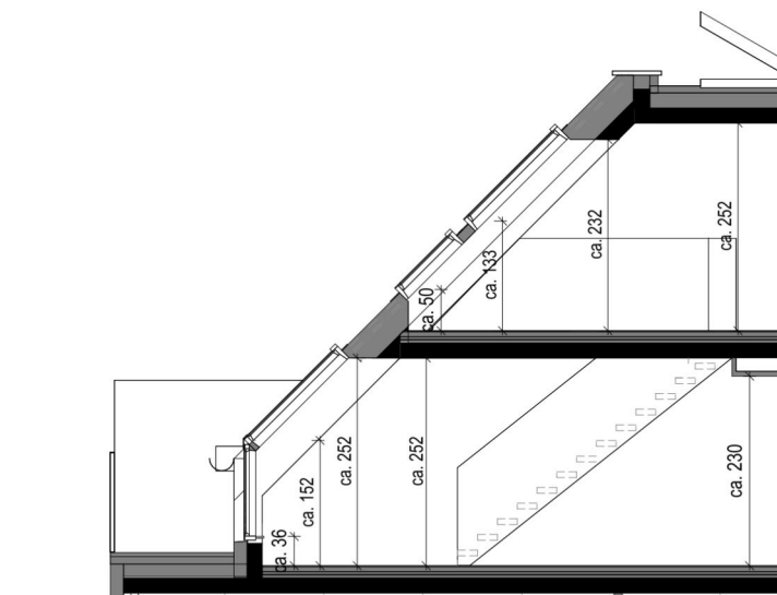
Schnitt 48.B
