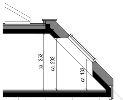
Schnitt 41.A
