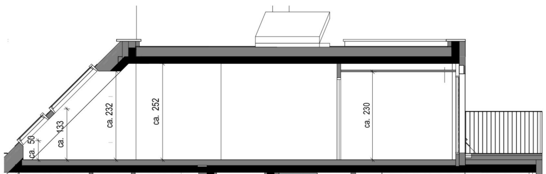
Schnitt 41.B
