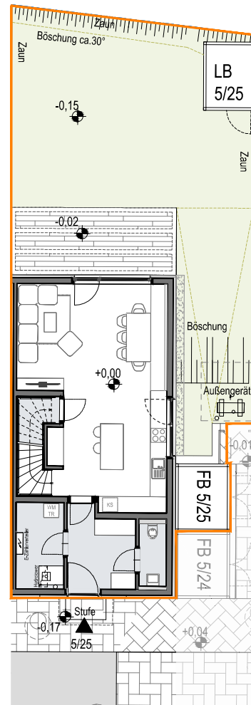
ERDGESCHOSS
