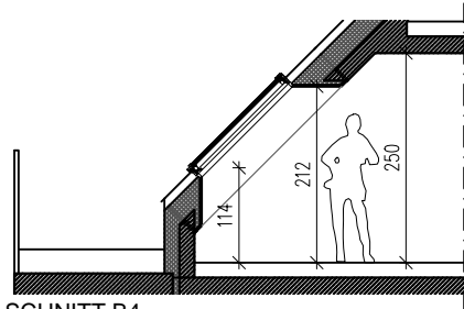
SCHNITT B4
