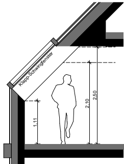
Schnitt 1
