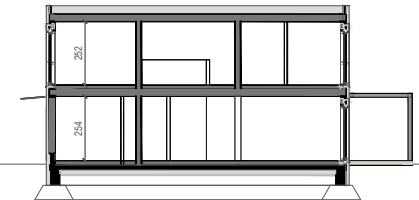
SCHEMATISCHER SCHNITT M 1:300
