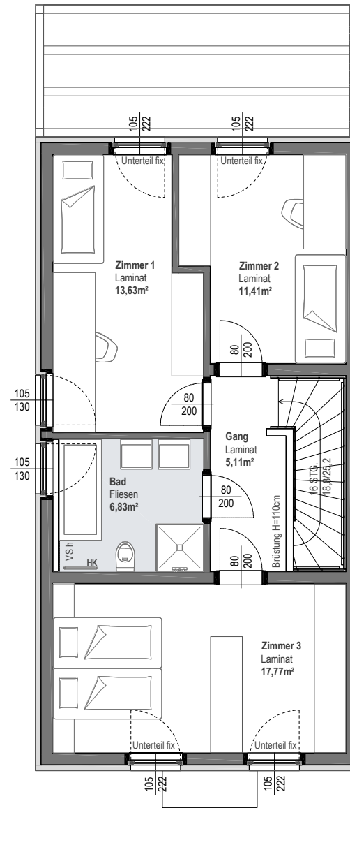
OBERGESCHOSS
