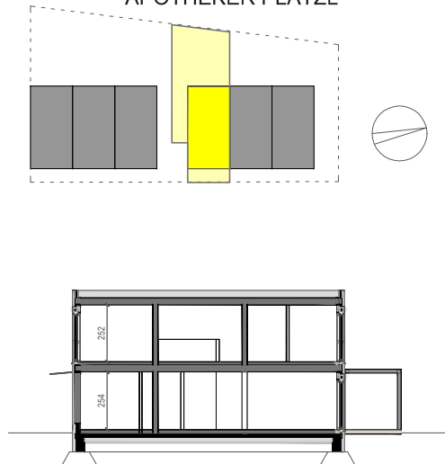
SCHEMATISCHER SCHNITT M 1:300
