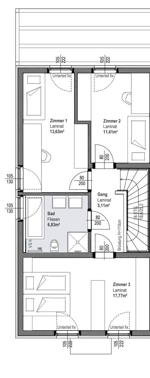
OBERGESCHOSS
