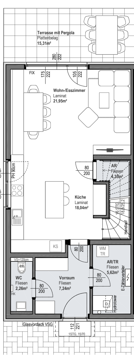
ERDGESCHOSS
