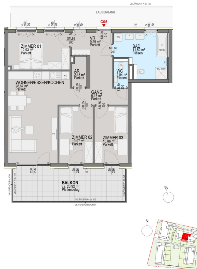
Grundriss 1. Obergeschoss:
