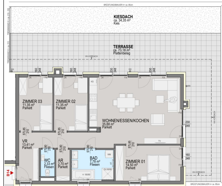
Grundriss Penthaus:
