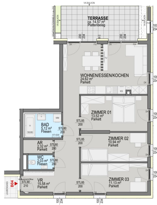
Grundriss Erdgeschoss:
