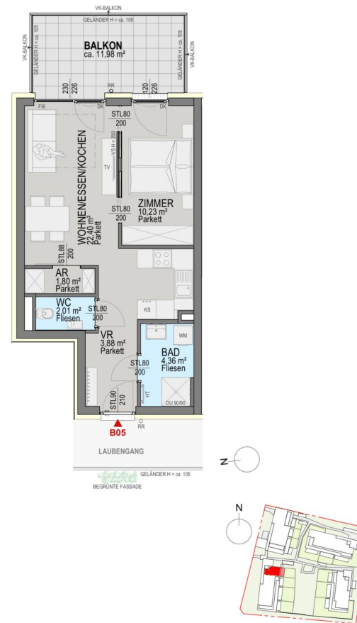
Grundriss 1. Obergeschoss:
