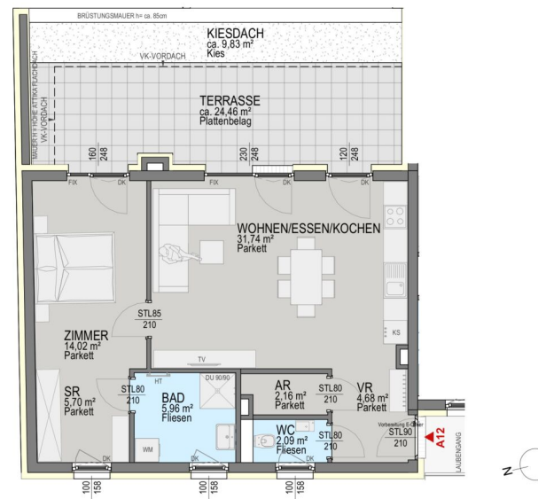
Grundriss Penthaus:
