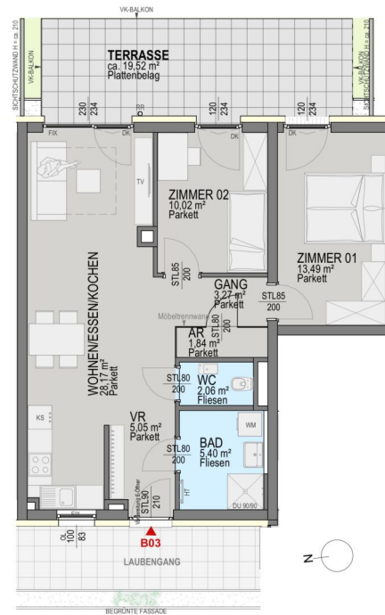
Grundriss Erdgeschoss:
