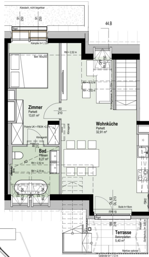
Grundriss Ebene 2 M 1 : 100
