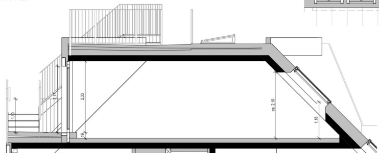
Schnitt 44.B M 1 : 100
