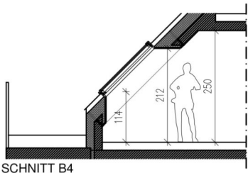
SCHNITT B4
