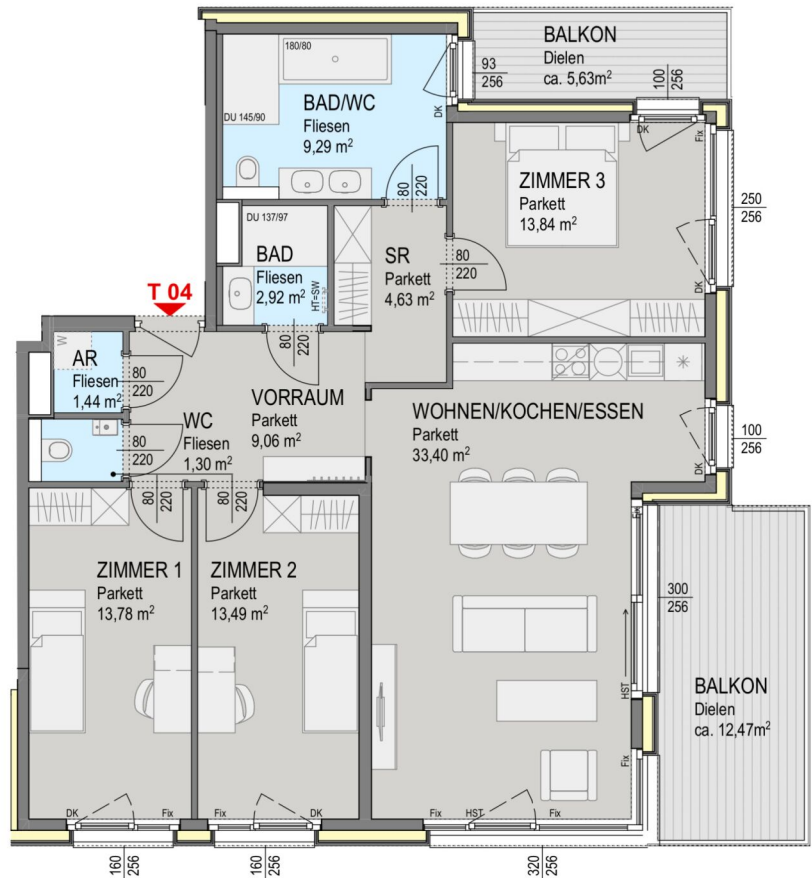
Grundriss Obergeschoss
