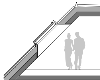
SCHNITT A
