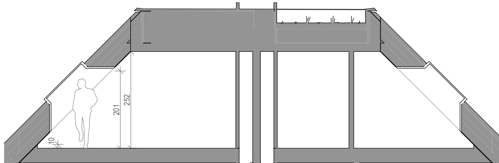
Schnitt 1-1
