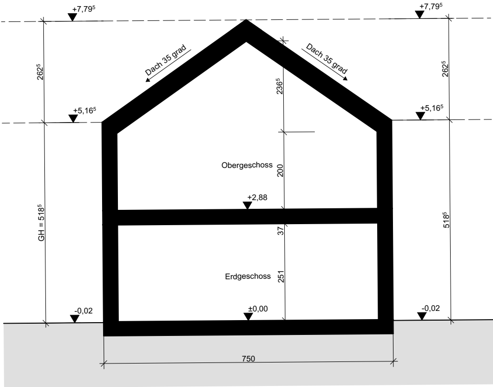
Schnitt 1:100
