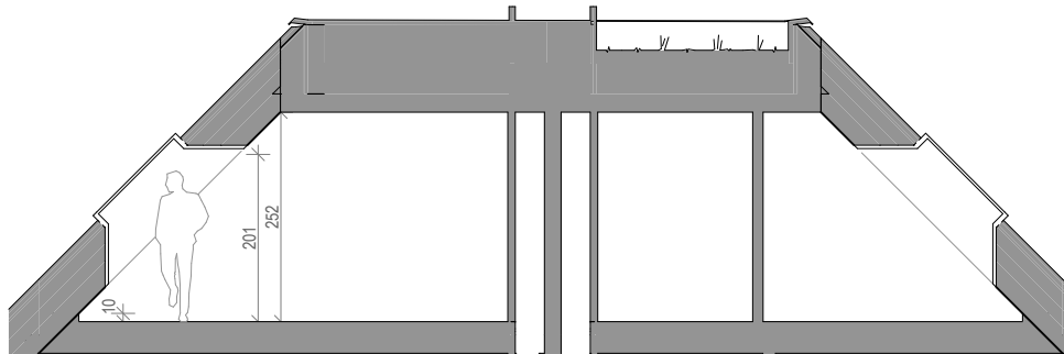
Schnitt 1-1
