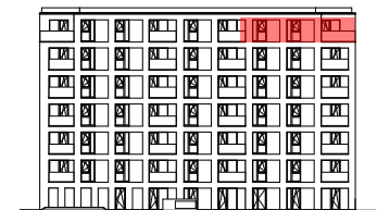
Ansicht Ost
