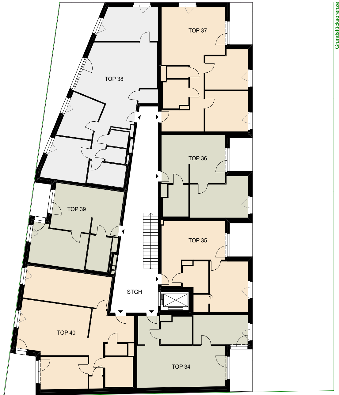
Übersichtsplan TOP 34-40 6. Obergeschoss
