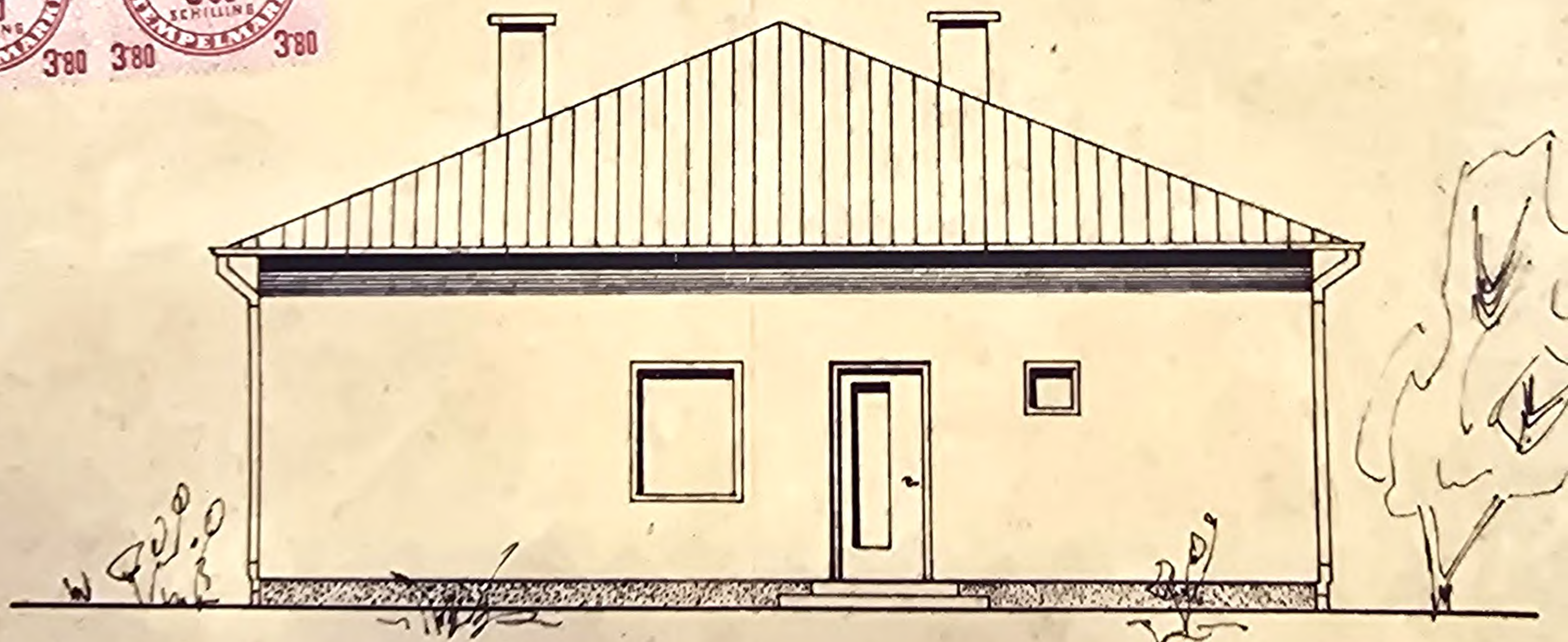
SÜDOSTANSICHT
