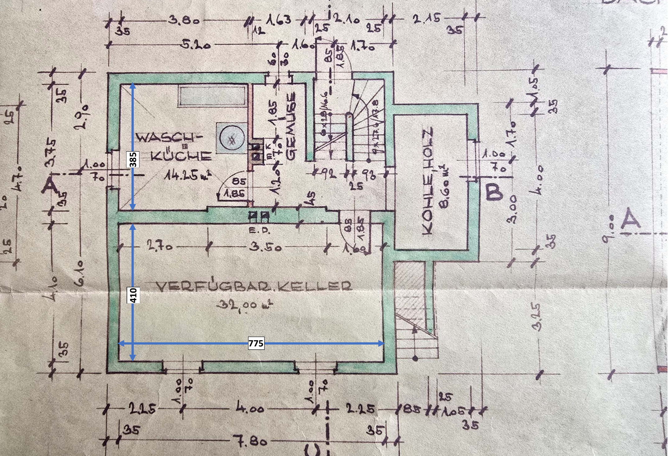
PLANSKIZZE Keller
