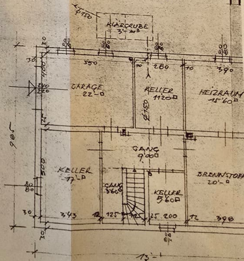
KELLERGESCHOSS.
