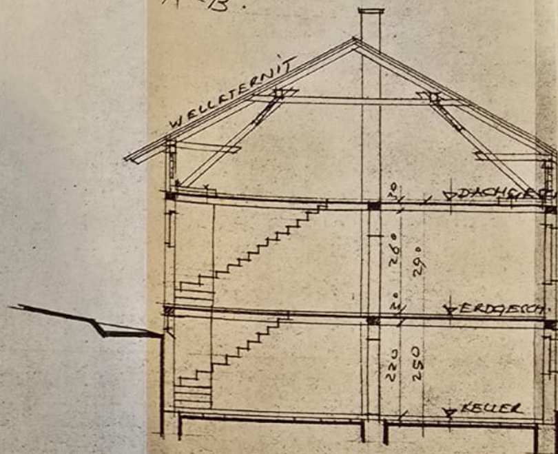
SCHNITT A-B.
