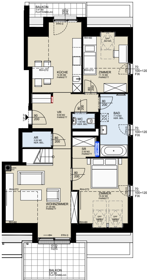
GRUNDRISS DACHGESCHOSS
