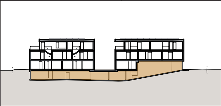
SCHNITT
