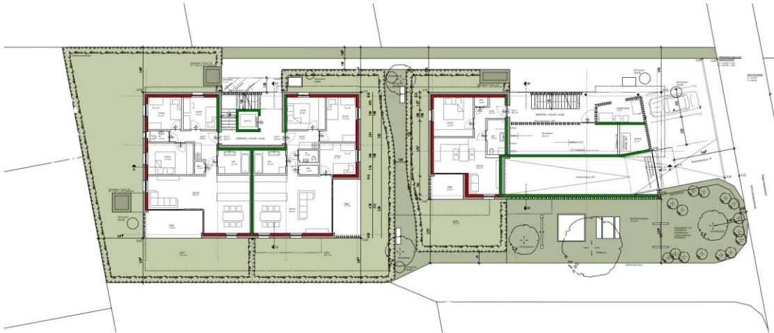
Auszug Lageplan
