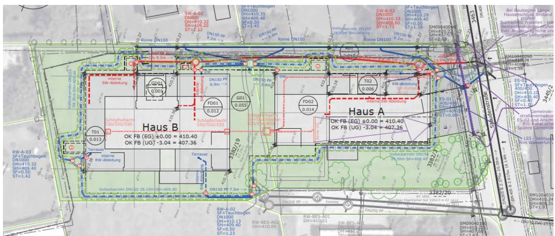
Auszug Entwässerungsplanung
